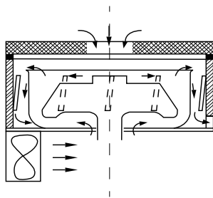
双风冷系统
