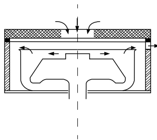
传统风冷系统
